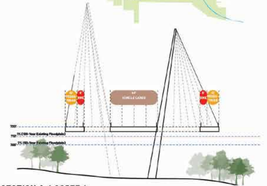
SECTION A / CORTE A
